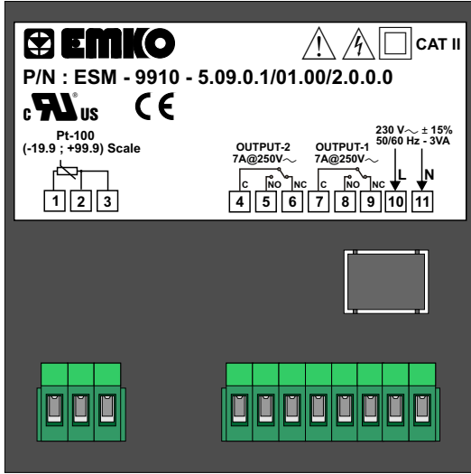
PT-100 (-19.9°C ; + 99.9°C) skala'lı cihazın arka kapak üzerindeki etiket görünümü
