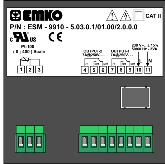
PT-100 (0°C ; 400°C) skala'lı cihazın arka kapak üzerindeki etiket görünümü
